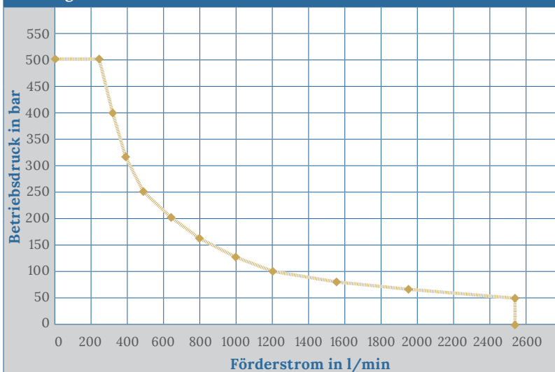
Leistungskurve SPL 106
